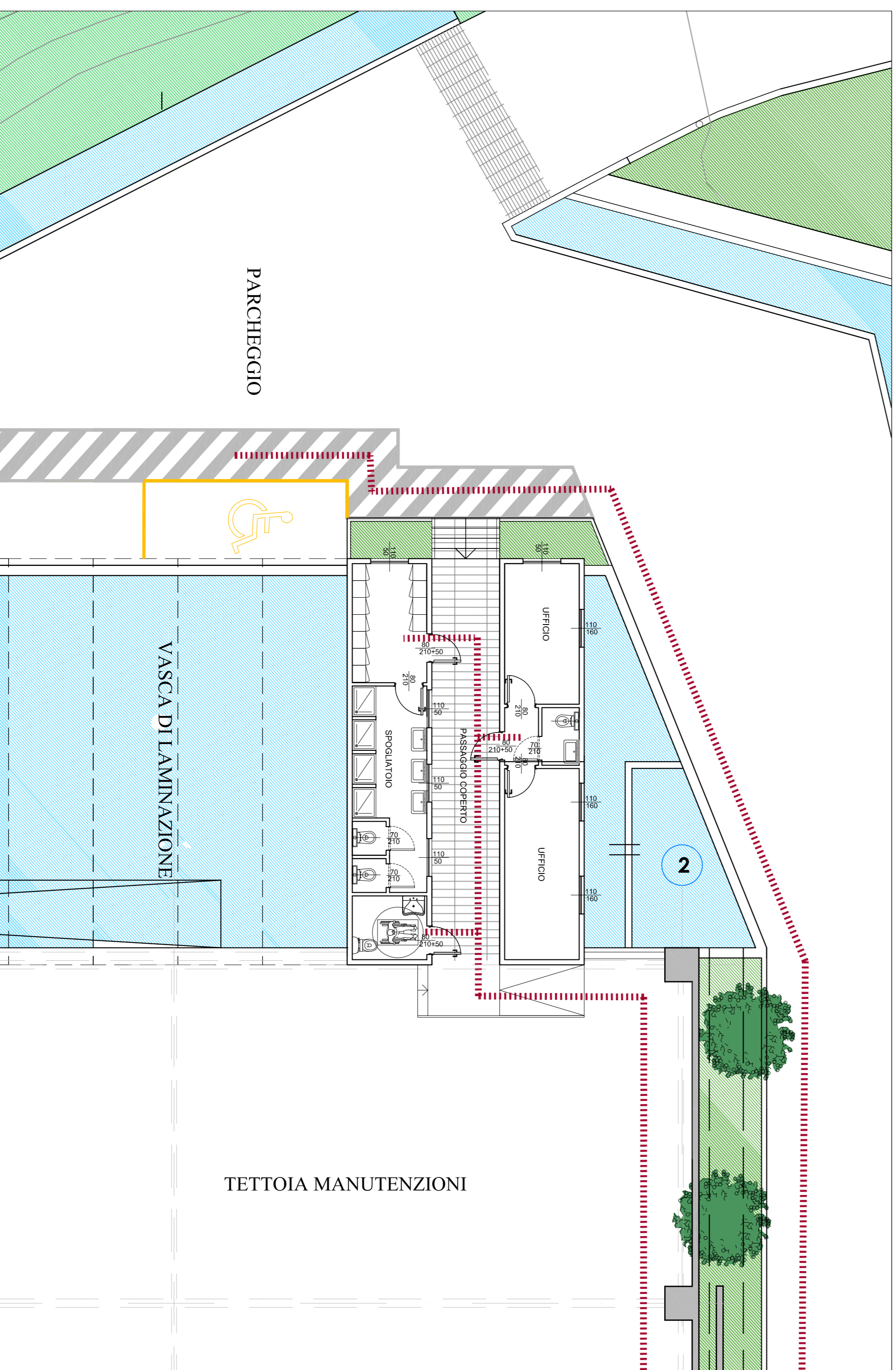
1 1/500 Planimetria Generale
