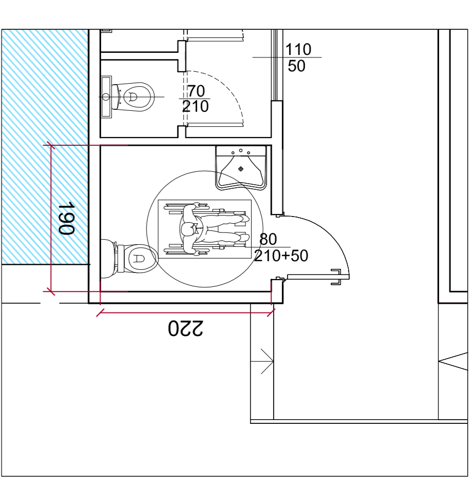
3 1/50 dett. bagno disabili
